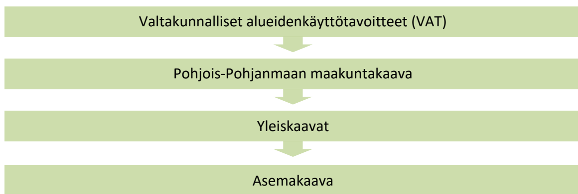
Kaavio 1. Kaavahierarkia
